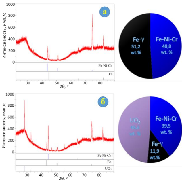
Рисунок 11 – Результаты РФА шлифов поперечного сечения образцов стали 12Х18Н10Т, выдержанных в солевой композиции LiCl-KCl – 2 мас. % UCl n . Доля UCl 3 : а) 5 %, б) 95%
