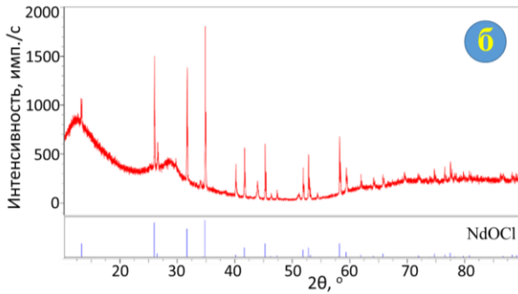
Рисунок 8 – Пример образования оксихлоридного слоя (расплав LiCl-KCl-2 мас. % NdCl 3 ) в окислительной газовой атмосфере в результате коррозионной выдержки образцов стали 12X18H10T течение 100 часов. а) МРСА, б) РФА
