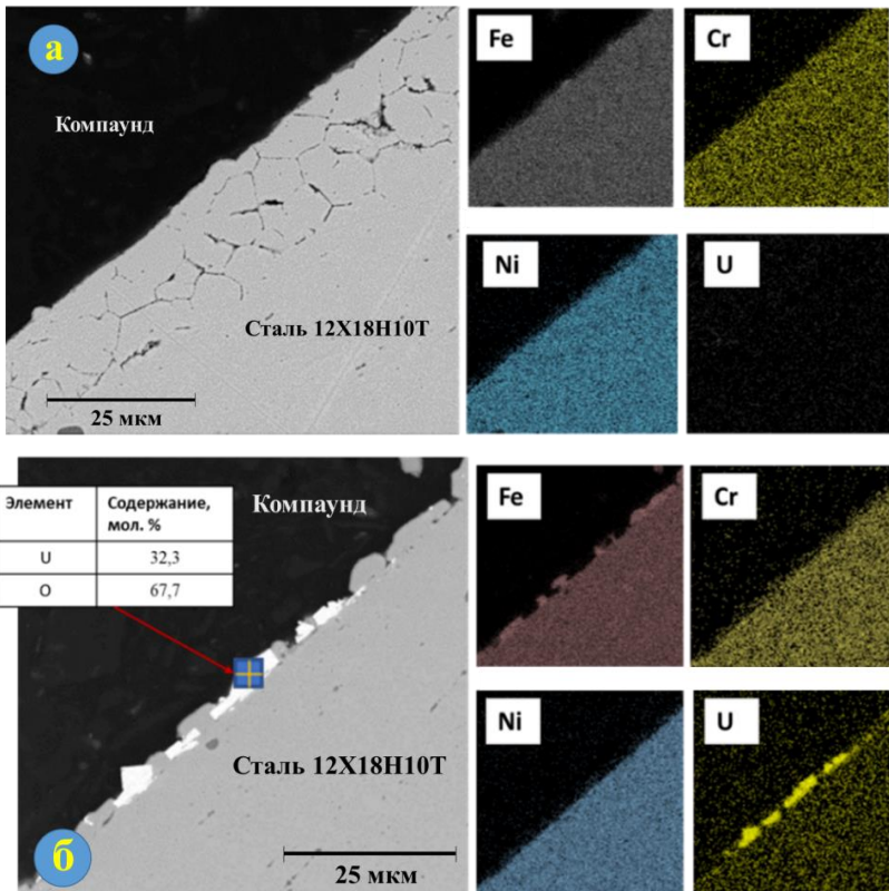
Рисунок 10 – Результаты МРСА шлифов поперечного сечения образцов стали 12X18Н10Т, выдержанных в солевой композиции LiCl-KCl – 2 мас. % UCl_n . Доля UCl_3 : а) 5 %, б) 95%
