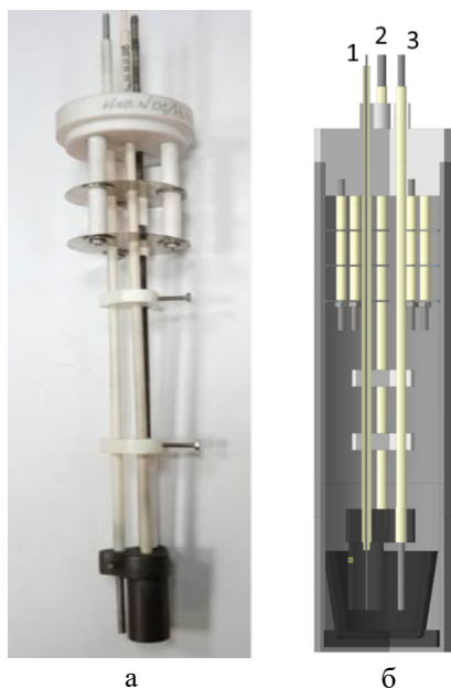
Рисунок 12 – Рабочая ячейка, используемая для проведения электрохимических измерений в расплаве \text{LiCl-KCl} с помощью литиевого динамического электрода сравнения:
