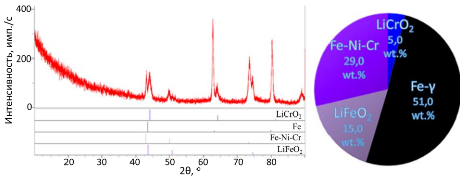
Рисунок 6 – Результаты РФА образцов стали после коррозионной выдержки в расплаве LiCl-KCl-2 мас. % Li 2 O
