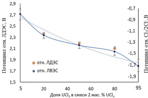
Рисунок 16 – Зависимость О-В потенциала среды от доли UCl 3 в расплаве LiCl-KCl-2 мас. % UCl n
