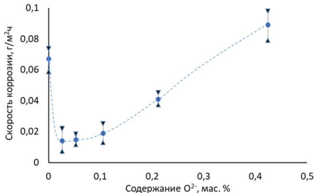
Рисунок 4 – Скорость коррозии стали 12X18H10T в зависимости от содержания анионов кислорода в расплаве LiCl- KCl-Li 2 O
