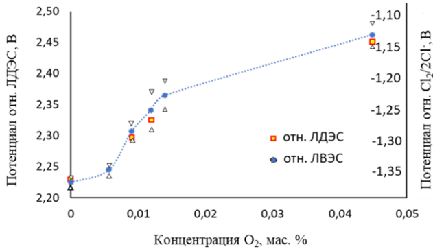
Рисунок 15 – Зависимость О-В потенциала среды от содержания молекулярного кислорода в расплаве LiCl-KCl
