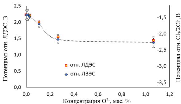
Рисунок 14 – Зависимость О-В потенциала среды от концентрации Li 2 O в расплаве LiCl-KCl (в пересчете на O 2- )
