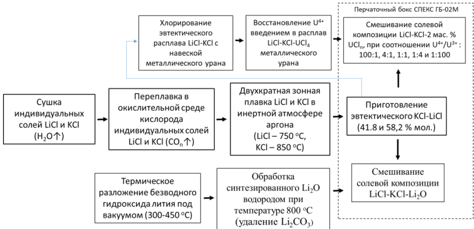
Рисунок 1 – Схема получения используемых солевых композиций на основе LiCl-KCl
