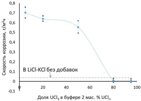
Рисунок 9 – Зависимость скорости коррозии образцов стали 12X18Н10Т, выдержанных в расплаве LiCl-KCl-2 мас. % UCl_n , от доли трехвалентного хлорида урана
