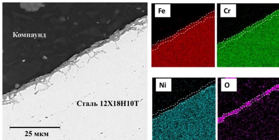
Рисунок 5 – Морфология образцов стали после коррозионной выдержки в расплаве LiCl-KCl-2 мас. % Li 2 O
