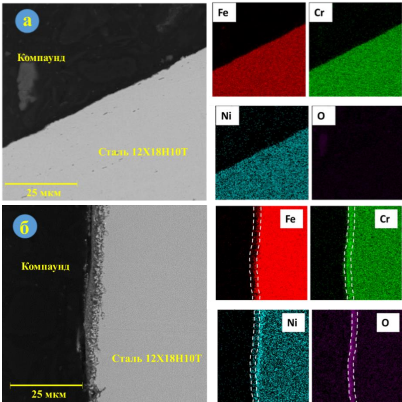
Рисунок 3 – Картинирование шлифа поперечного сечения образца 12X18H10T, выдержанного в расплаве LiCl-KCl в течение 100 часов. Газовая атмосфера над расплавом: а) Ar, б) Ar + 20 об. % O 2
